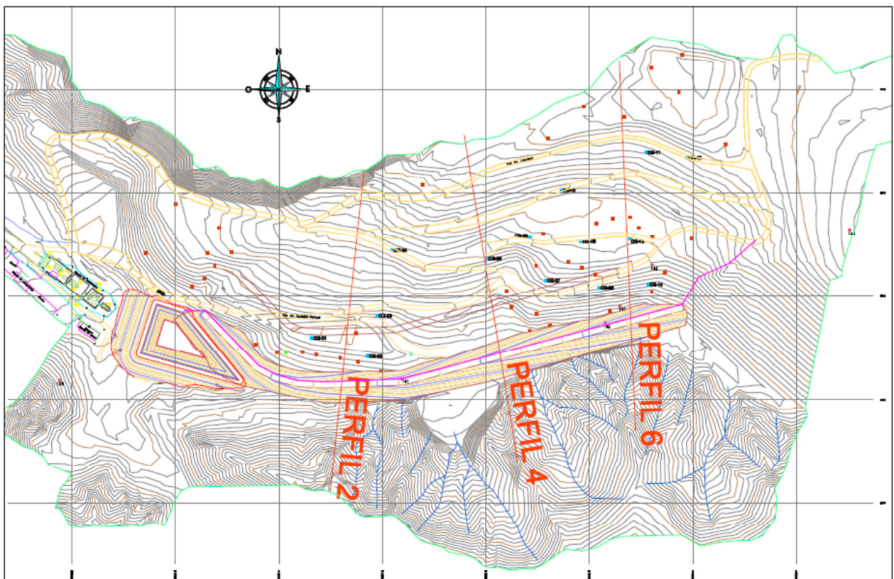
Figura 2. Dique de contención inferior – Vista en planta
