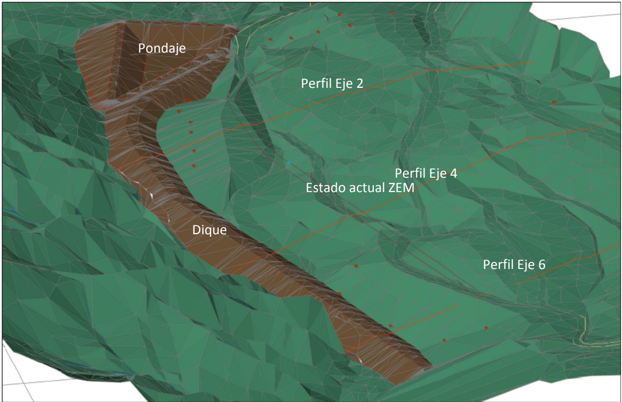
Figura 4. Perfiles de secciones 2, 4 y 6, según se definió por geotecnia
