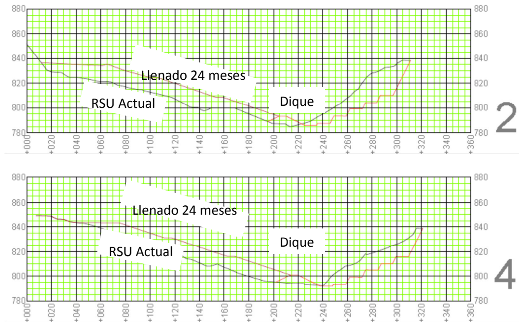
Figura 4. Perfiles de secciones 2, 4 y 6, según se definió por geotecnia
